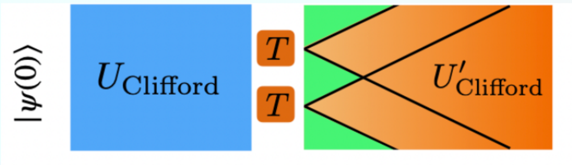
SciPost Phys. 9, 087 (2020)
