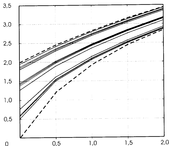
Slika 3.5: Fononski spektar jako perturbovanog filma
