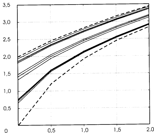
Slika 3.4: Fononski spektar jače perturbovanog filma
