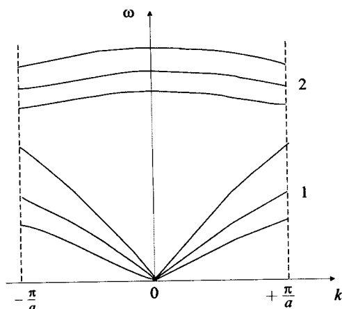
Slika 2.3: Akustičke (1) i optičke (2) fononske grane
