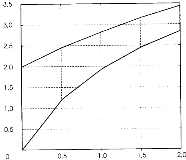
Slika 2.2: Fononski spektar balk uzorka
