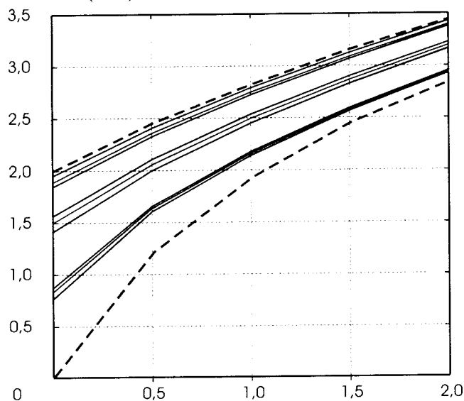
Slika 3.3: Fononski spektar slaboperturbovanog filma
